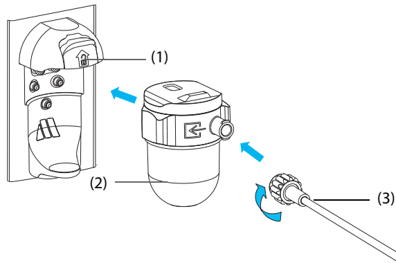
(1) Prise du piège à eau (2) Piège à eau DRYLINE II (3) Tubulure d'échantillonnage de gaz
